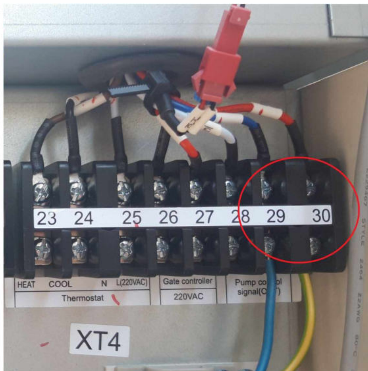
Listwa zaciskowa XT4
