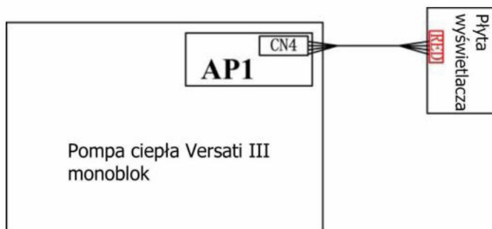
Schemat podłączenia sterownika przewodowego
