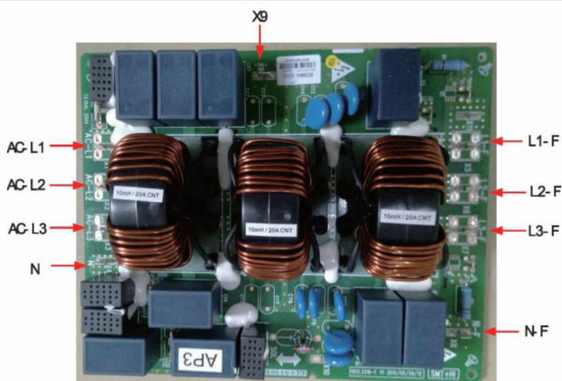
Płyta sterowania AP 3
