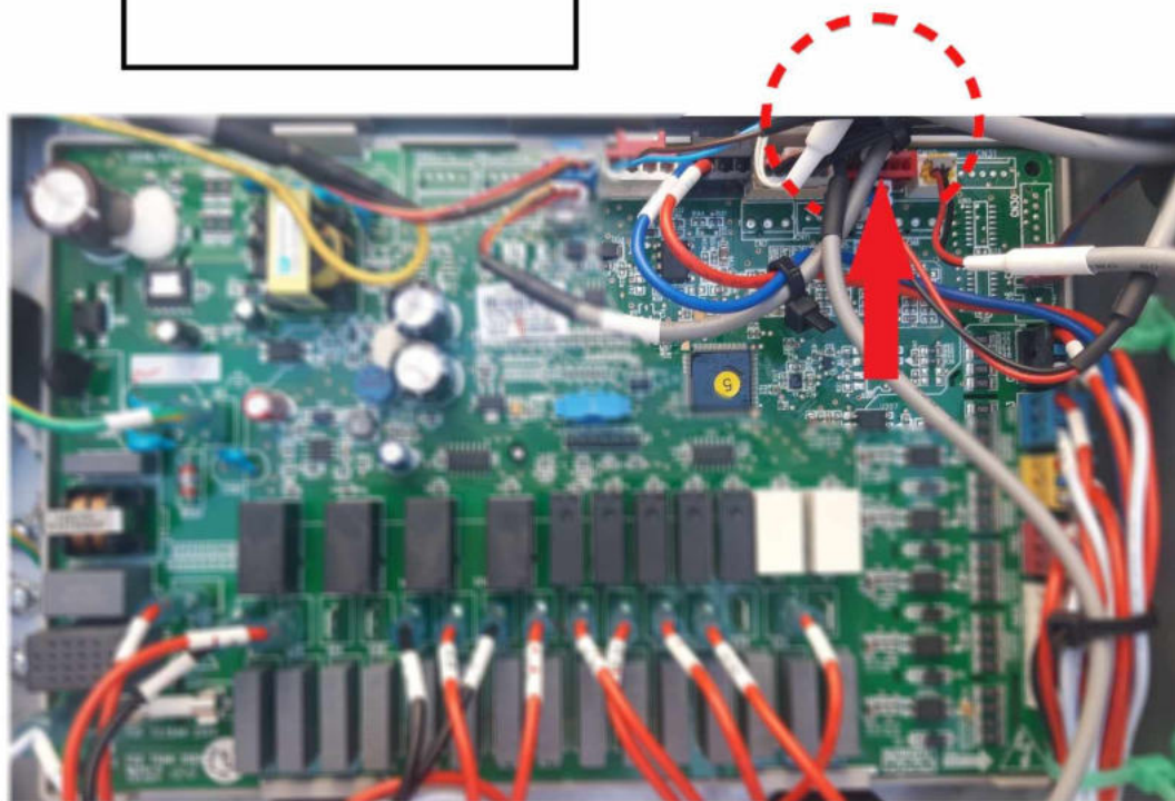
Miejsce mocowania wtyczki na płycie głównej dla opcjonalnego czujnika wody
