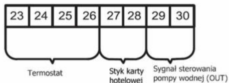
Listwa zaciskowa XT4
