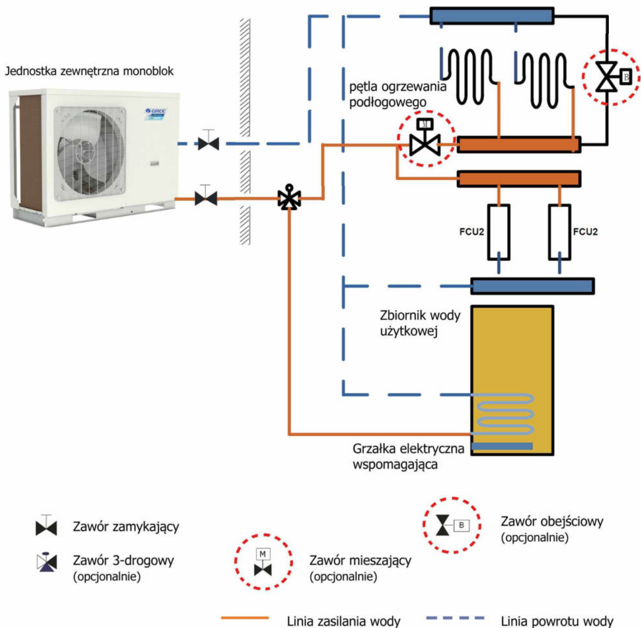
Przykład 3: Podłączenie zbiornika wody użytkowej, pętli ogrzewania podłogowego i klimakonwektorów FCU
