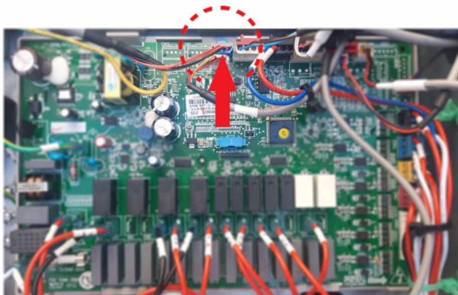
Schemat podłączenia sterownika przewodowego
