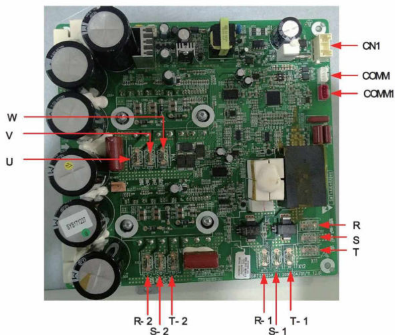
Płyta sterowania AP 4
